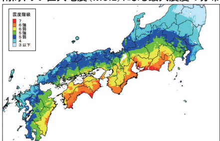
南海トラフ巨大地震(M9.1)による最大震度の分布
