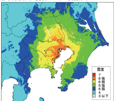
都心南部直下地震(M7.3)の震度分布
